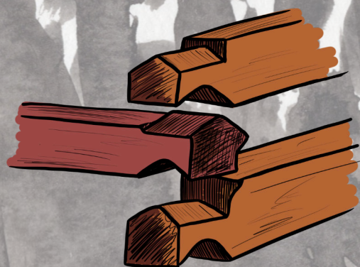
ASSEMBLAGE EN V
