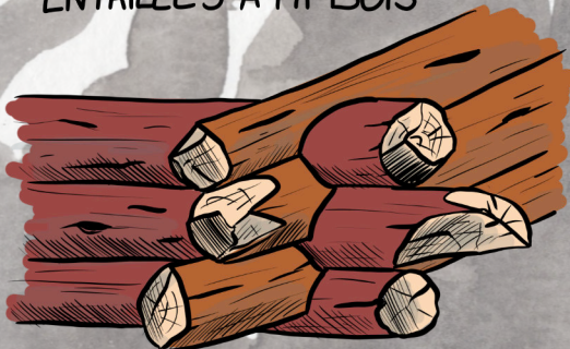
ASSEMBLAGE À ENTAILLES À MI-BOIS
